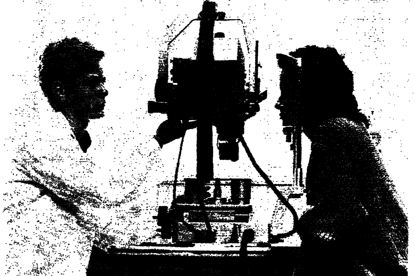
Mit der Scheinplugh-Kamera können Trübungen der Augenlinse frühzeitig erkannt werden. Ihr Funktionsprinzip: Indem sich die Ebenen des einfallenden Lichts, des Objektivs und der Abbildung in einem einzigen Punkt schneiden, wird eine tiefenschärfte Abbildung eines schräg zur Kamera stehenden Objektes erreicht (s. Foto links) FOTO POLY-PRESS
